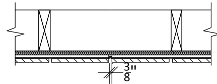
Fig.5 - Espaciado de Juntas de Paneles Verticales
